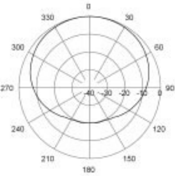
H-Plane | 1500 MHz
