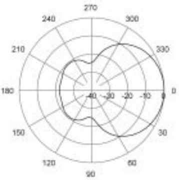
E-Plane | 1500 MHz
